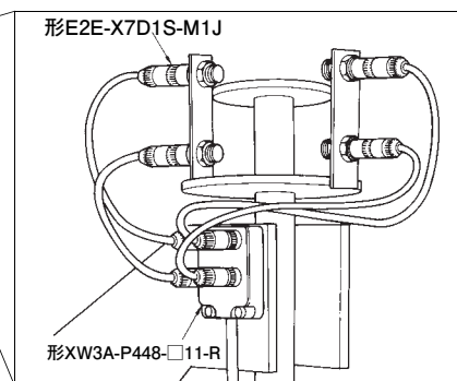
形XW3A周辺の配線イメージ
