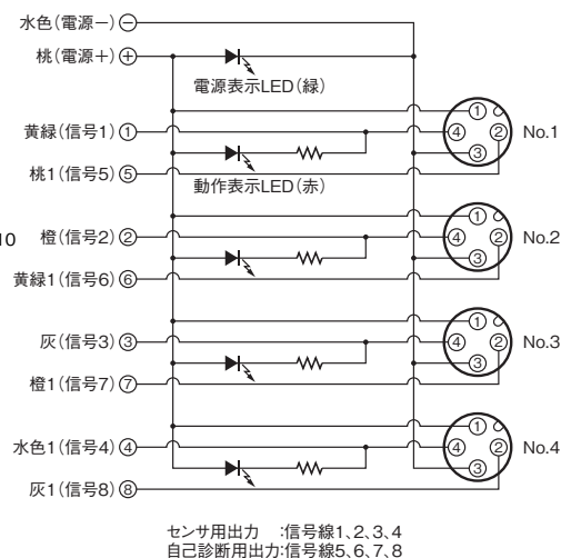
回路図
