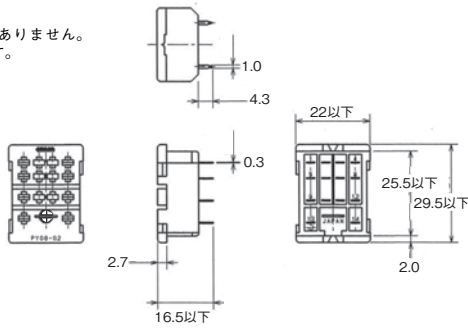
端子配置/内部接続図
