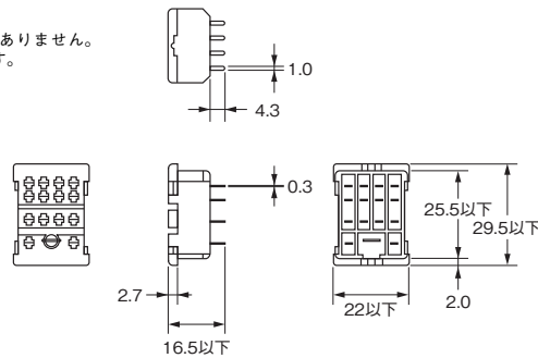
端子配置/内部接続図
