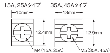
出力端子部(单相タイプ)
