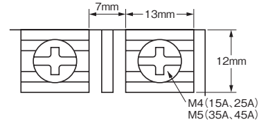
出力端子部(单相タイプ)
