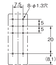
取り付け穴加工寸法 (BOTTOM VIEW)
