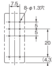
取り付け穴加工寸法 (BOTTOM VIEW)
