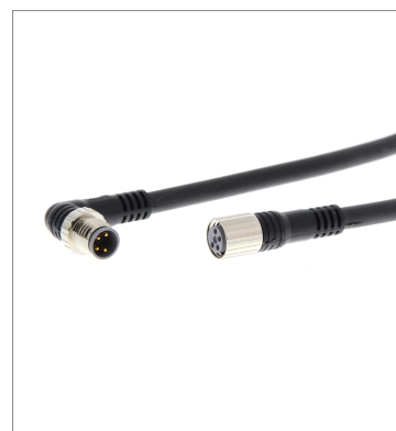
丸型防水コネクタ XS3W-M423-401-R
