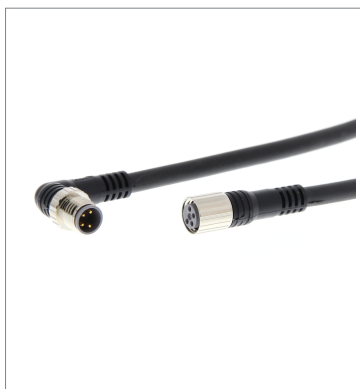
丸型防水コネクタ XS3W-M423-402-PR
