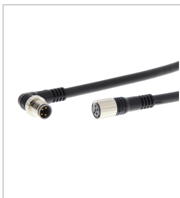
丸型防水コネクタ XS3W-M423-401-PR
