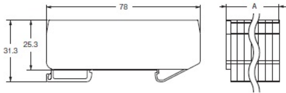
A寸法
