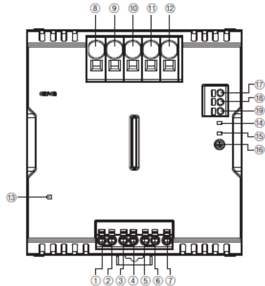
形S8VK-WB960□□
