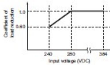
DC input
