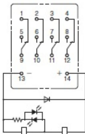
形MY4(Z)IN-D2(S) (DC仕様のみ)
