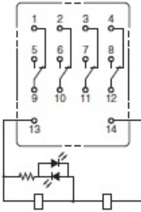
形MY4(Z)IN(S) (DC仕様)
