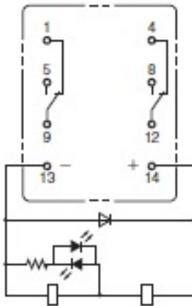
形MY2IN-D2(S) (DC仕様のみ)
