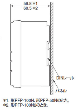
DINレール取り付けの場合
