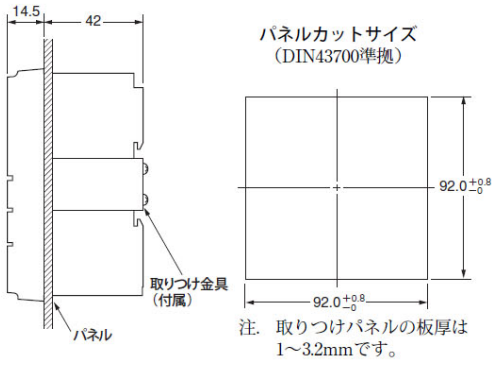
埋込み取り付けの場合
