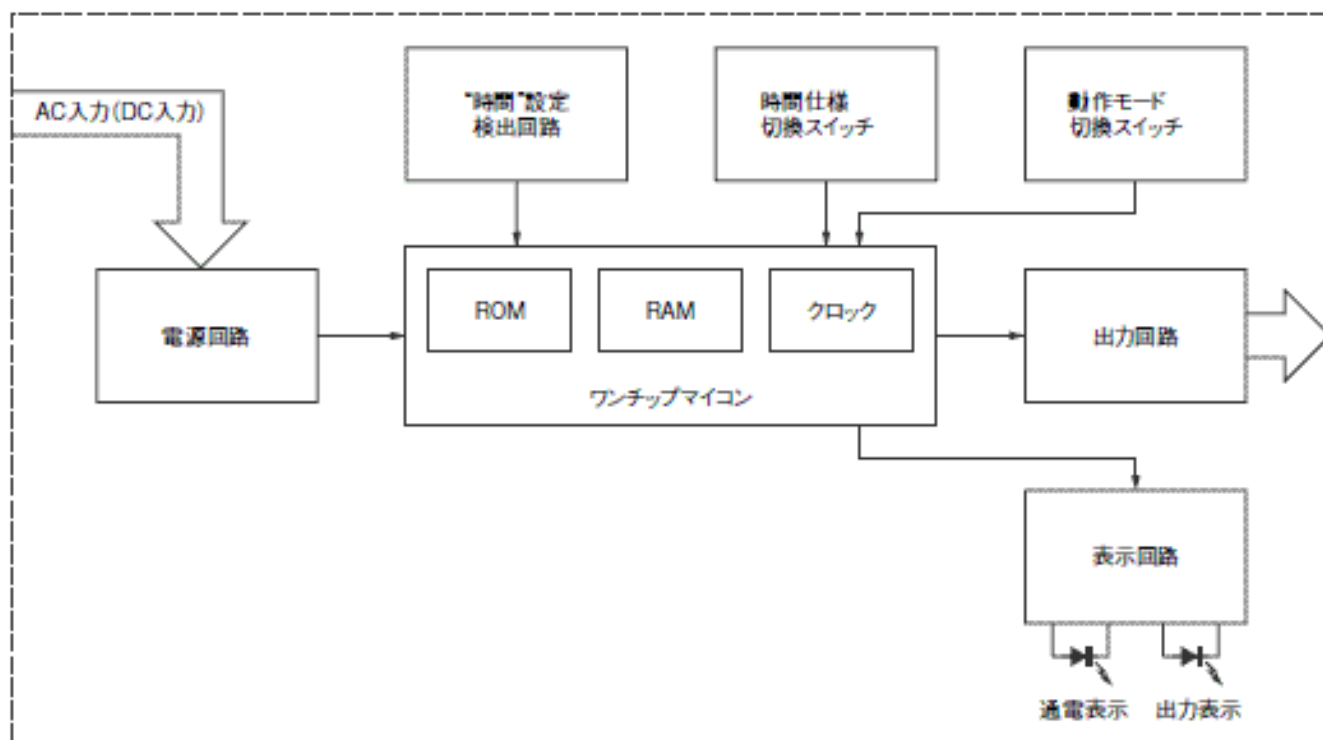
内部接続図
