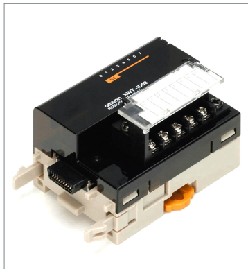
リモートI/Oターミナル XWT-ID08
