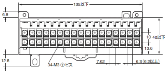
端子ブロック (増設端子なし)
