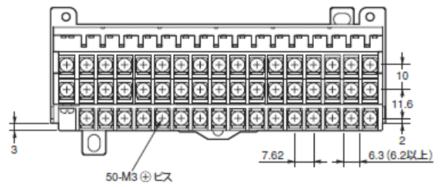
端子ブロック (増設端子台接続時)
