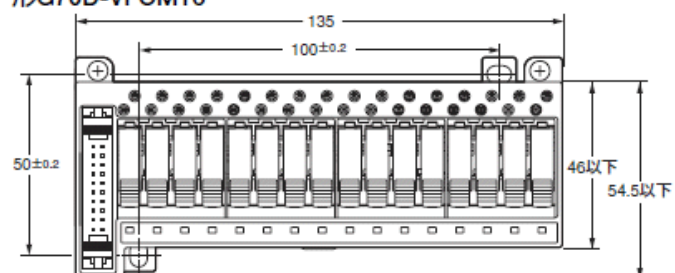
形G70D-VSOC16 形G70D-VFOM16
