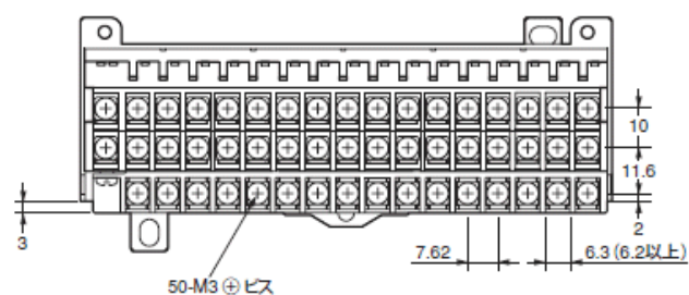
端子ブロック (増設端子台接続時)
