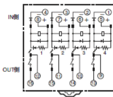
端子配置／内部接続図 (TOP VIEW)
