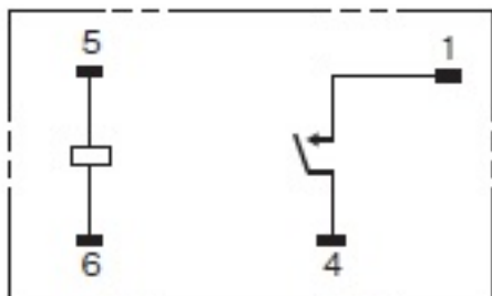
端子配置/内部接続図 (BOTTOM VIEW)
