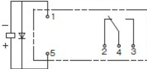
形G2R-1-SD (DC仕様)
