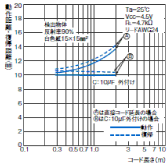
形EE-SPY□□□
