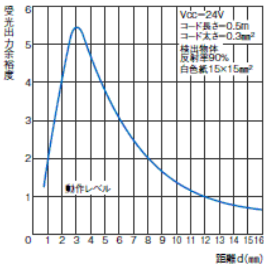
形EE-SPY□□□
