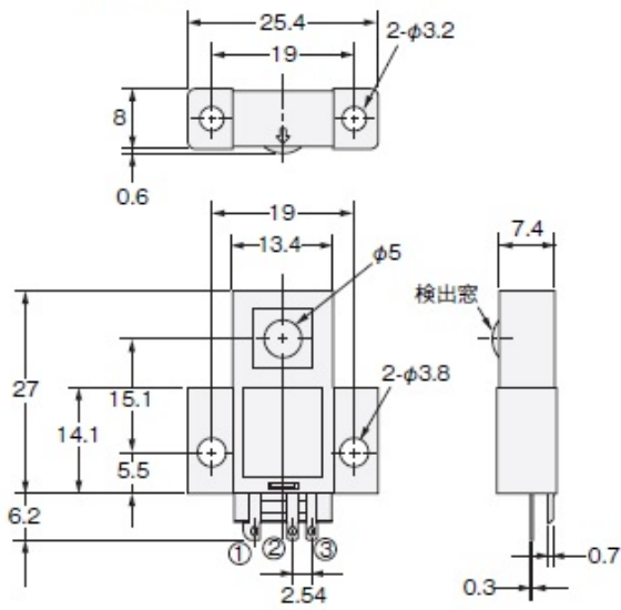
投光器 (形EE-SPWL□11)
