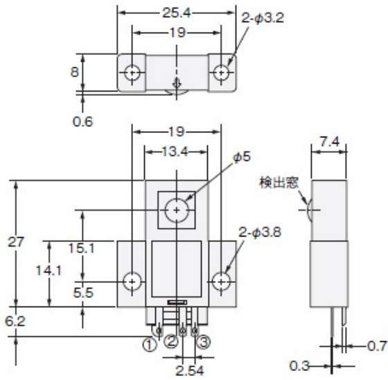
投光器 (形EE-SPWL□11)
