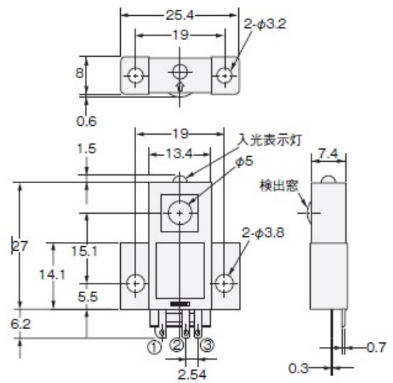
受光器 (形EE-SPWD□11)
