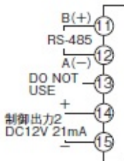
形E5CN-H□□□□□03
