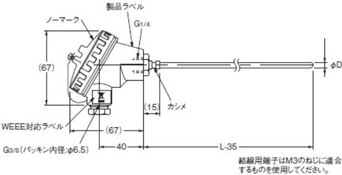
●形E52-P□C-N 外形寸法 (単位: mm、ただしLはcm)
