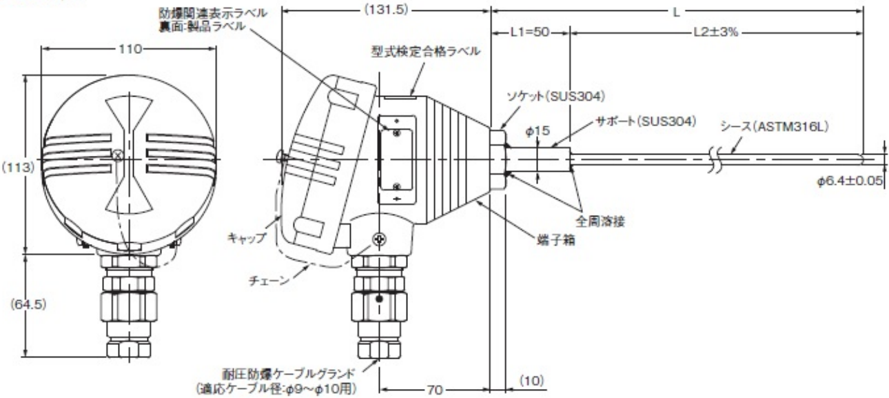
●形E52-CA□□C-N-6 外形寸法
