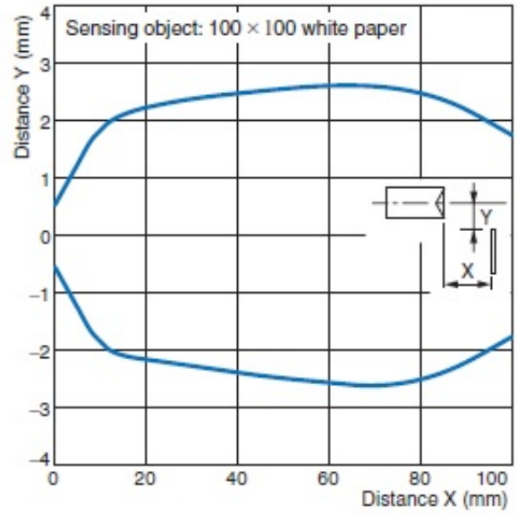
E3ZM-LS□1H(LS□6H), Left to Right
