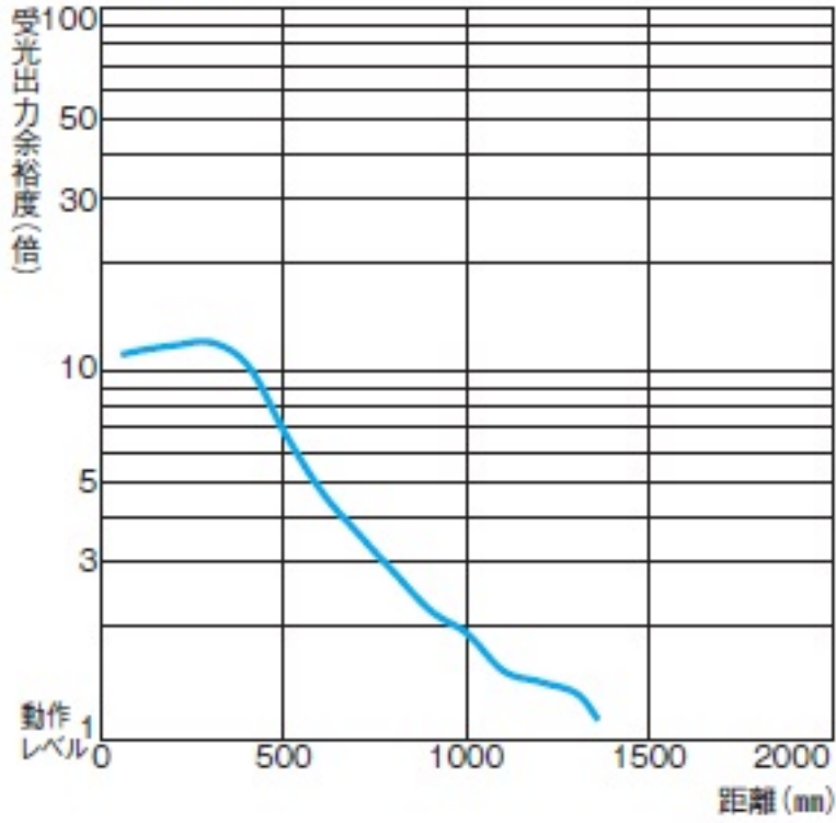
形E3T-ST2□F
