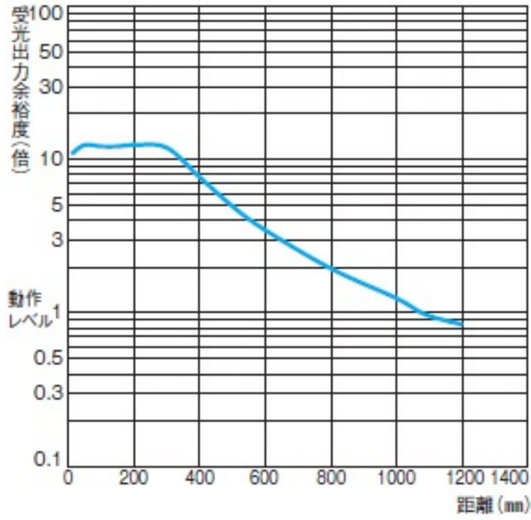
形E3T-FT2□F
