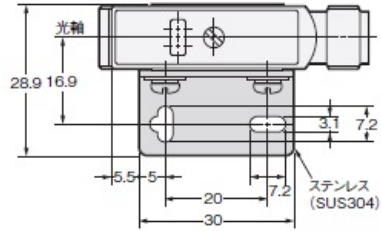
取り付け金具装着時
