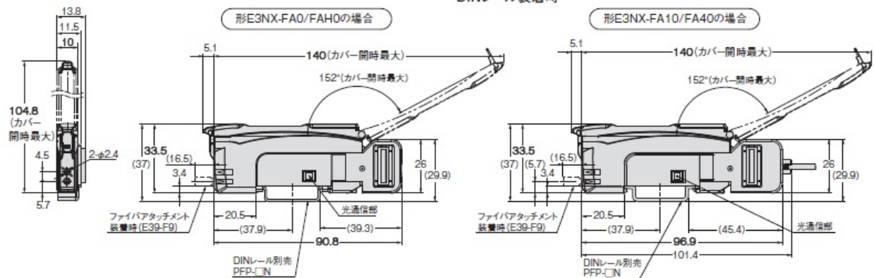
DINレール装着時
