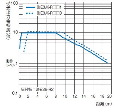
形E3JK-R□□1+形E39-R2/ 形E3JK-R□□3+形E39-R2
