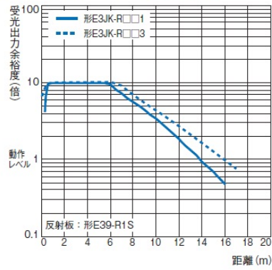
形E3JK-R□□1+形E39-R1S/ 形E3JK-R□□3+形E39-R1S
