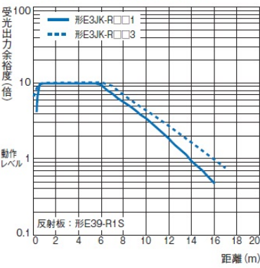
形E3JK-R□□1+形E39-R1S/ 形E3JK-R□□3+形E39-R1S
