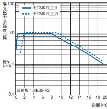
形E3JK-R□□1+形E39-R2/ 形E3JK-R□□3+形E39-R2
