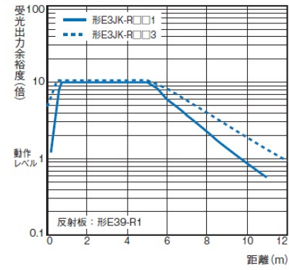
形E3JK-R□□1+形E39-R1/ 形E3JK-R□□3+形E39-R1
