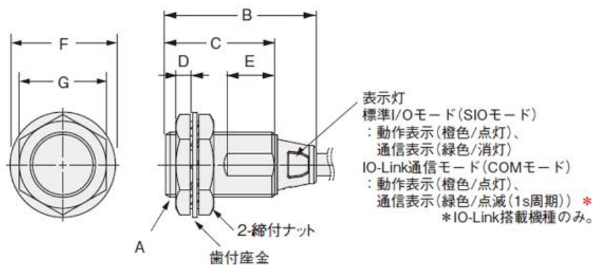
外形図
