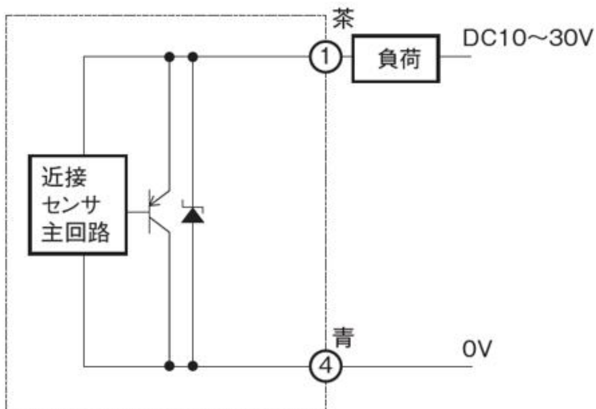
出力段回路図
