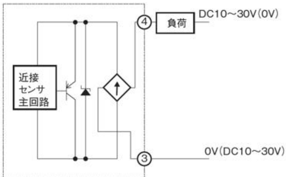
出力段回路図
