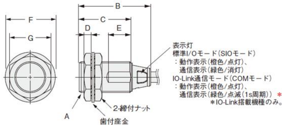
外形図
