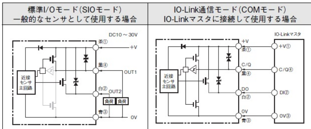
出力段回路図
