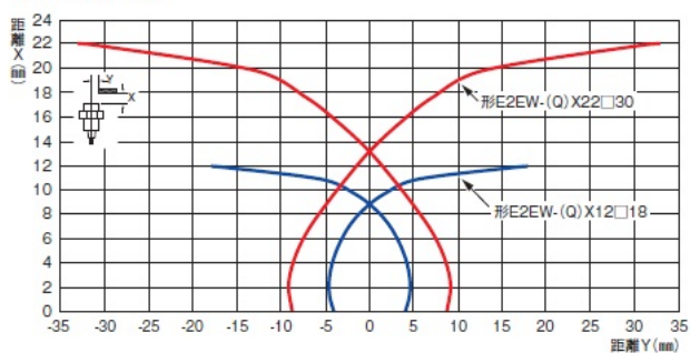
検出物体：鉄
