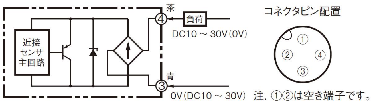
出力段回路図
