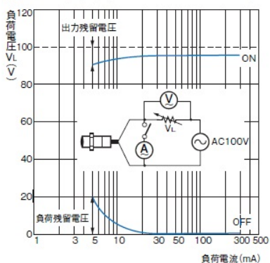
形E2E-X□Y□ AC100Vの時
