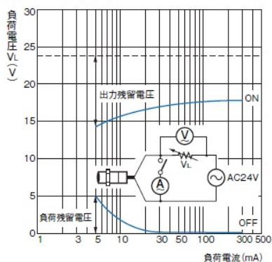
形E2E-X□Y□ AC24Vの時
