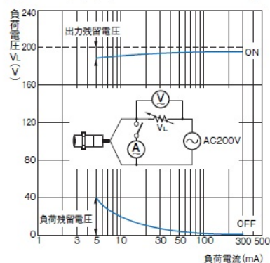
形E2E-X□Y□ AC200Vの時
