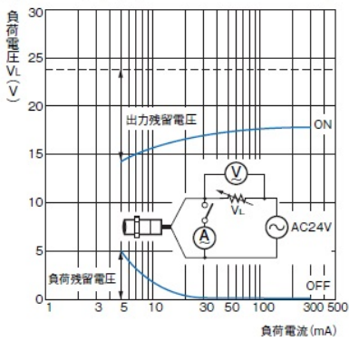
形E2E-X□Y□ AC24Vの時
