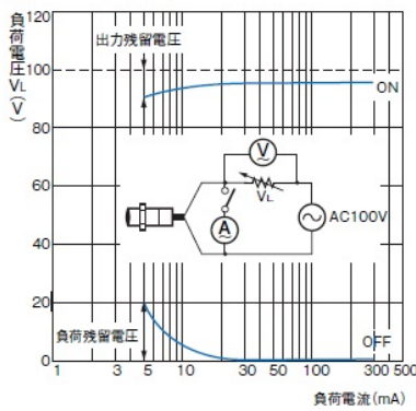
形E2E-X□Y□ AC100Vの時
