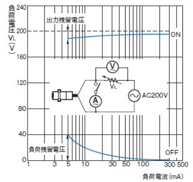
形E2E-X□Y□ AC200Vの時
