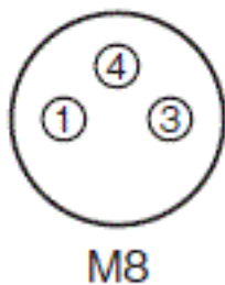
コネクタピン配置
