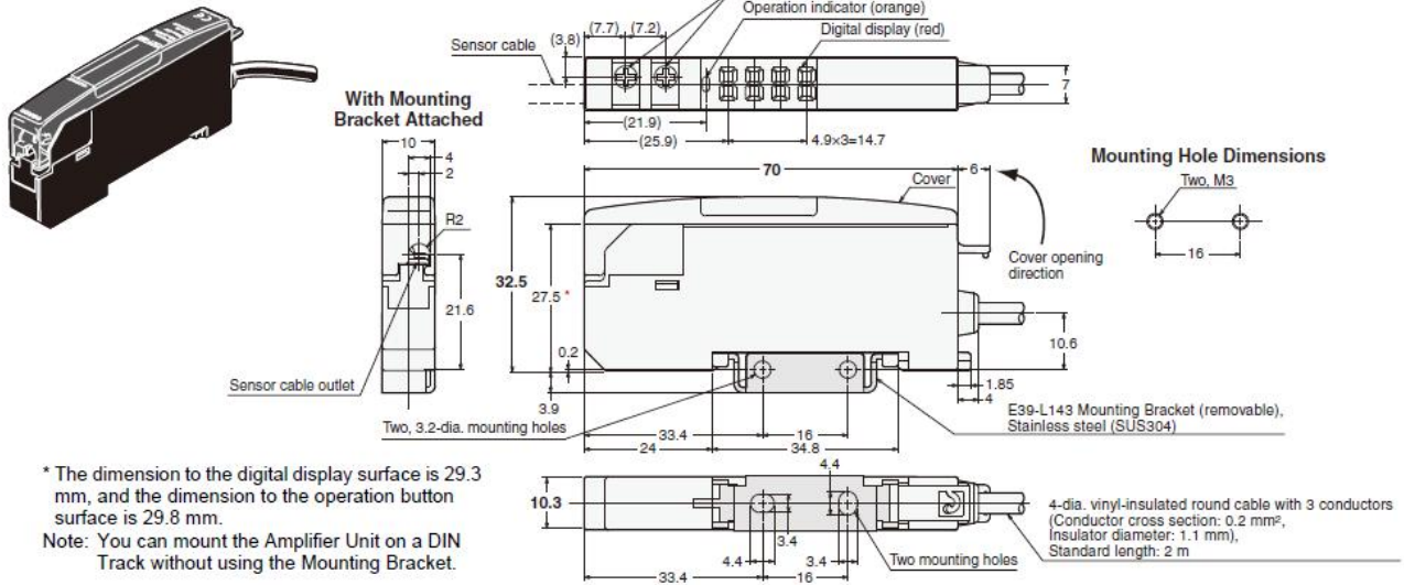
E2CY-SD11 E2CY-SD41
