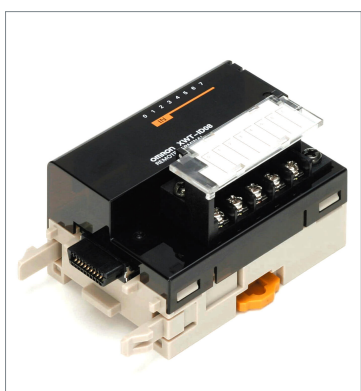
リモートI/Oターミナル
