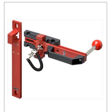
スライドキーユニット D4SL-NSK10-LKH
