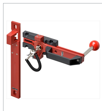
スライドキーユニット D4SL-NSK10-LKH
