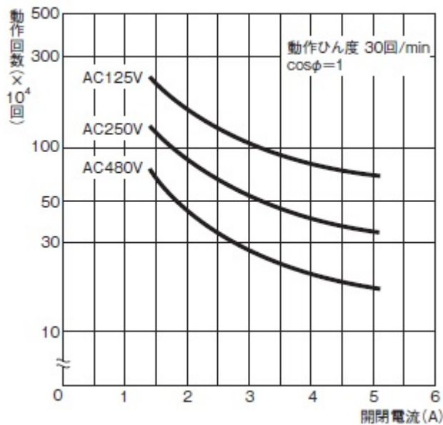
電氣的耐久曲線/4回路双断形
