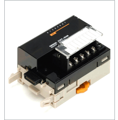
リモートI/Oターミナル XWT-OD08
