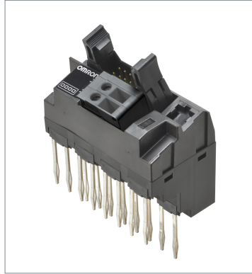
PLCインターフェースユニット P2RVC-8ST-O-7-1
