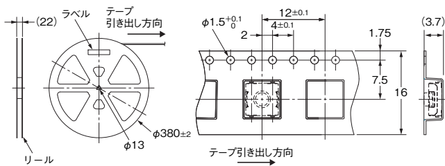
100個梱包用リール (形B3SL-100□P-R100)
