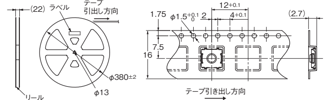
100個梱包用リール (形B3SE-1002P-R100)
